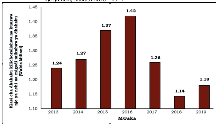
Kielelezo Na.3: Kiasi cha dhahabu kilichozalishwa katika migodi mikubwa na kuuzwa nje ya nchi, mwaka 2013 - 2019
