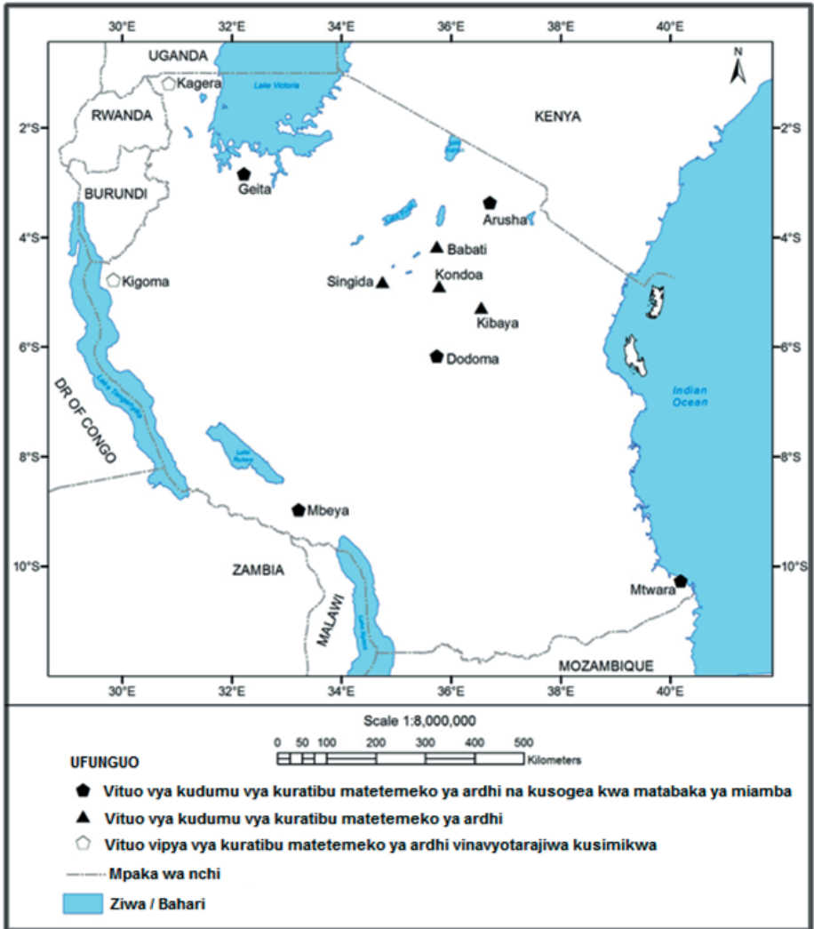
Kielelezo Na.5: Ramani inayoonesha vituo vya kupimia mitetemo ya ardhi
