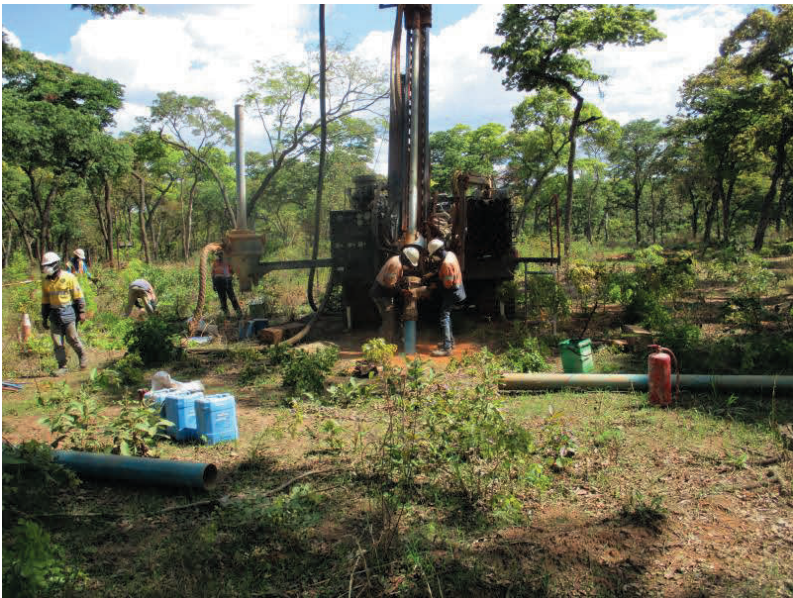
Picha Na. 21: Wataalam wa STAMICO wakiwa katika Shughuli za Uchorongaji
